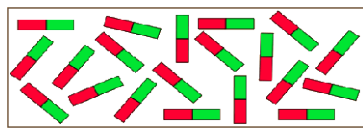
ungeordnete Elementarmagnete
